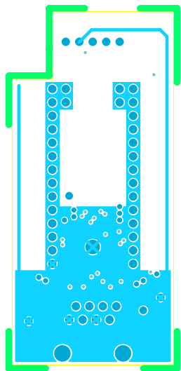
PDCR-9297 REV *A LAYER 2 GND
